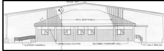
Elevation
